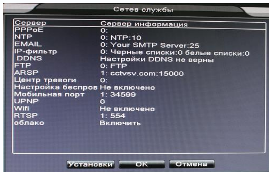
Рис. 4.18 Сетевые сервисы
